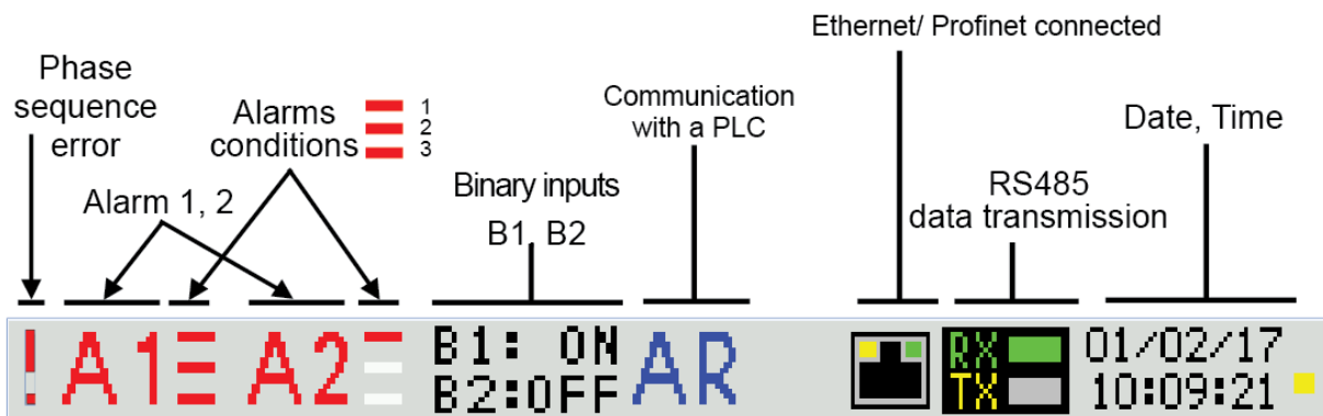
Fig.10. Information bar
