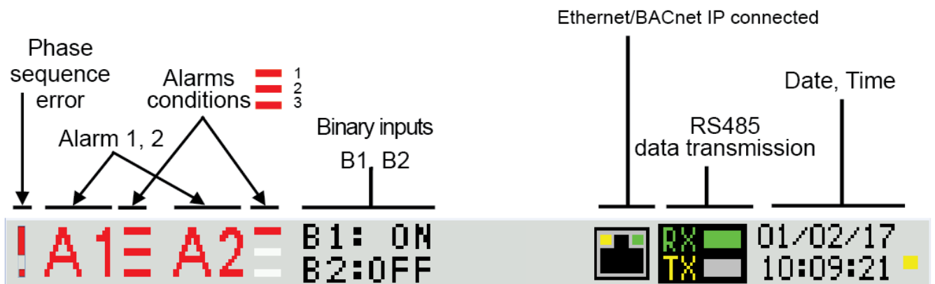
Fig. 10. Information bar
