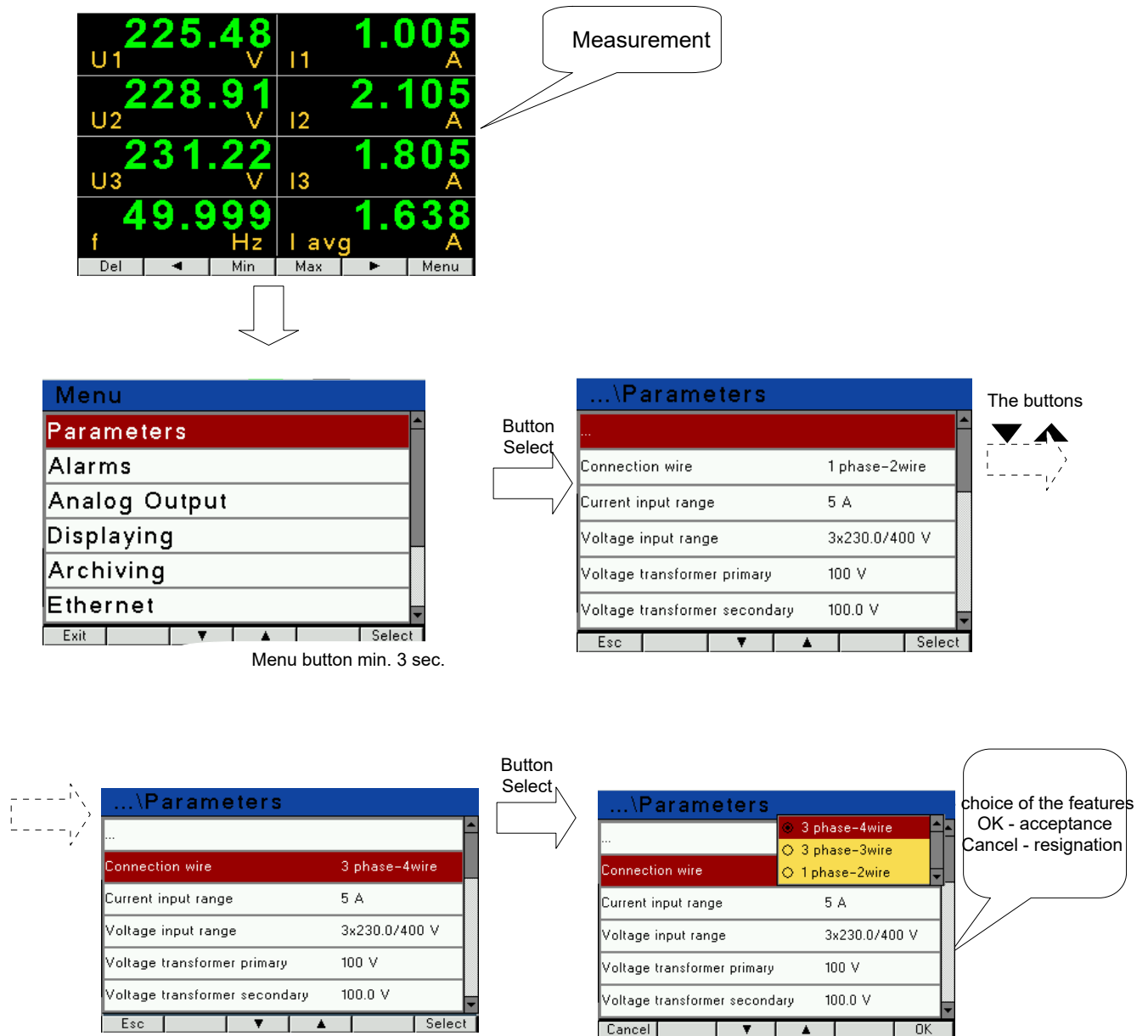
Fig. 19. Screens of Parameters mode
